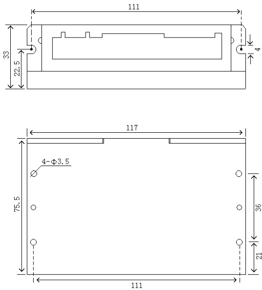
安装尺寸（单位：mm）
