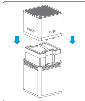
⑥ 装入机器上半部分。
